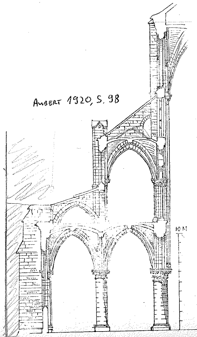
Fig. 15. — Notre-Dame de Paris. Coupe sur le chœur. Restitution de l'état au XII e siècle.
