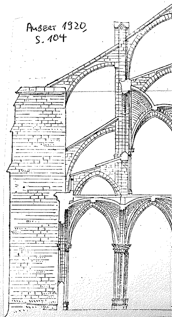
— Notre-Dame de Paris. Coupe sur la nef. Restitution de l'état au XII e siècle.
