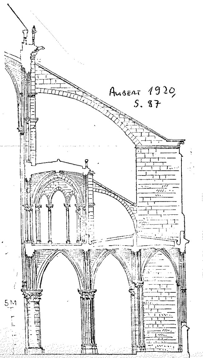
Fig. 10. — Notre-Dame de Paris. Coupe sur la nef, avant la restauration de Viollet-le-Duc.
